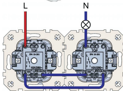
Układ dwóch łączników schodowych
